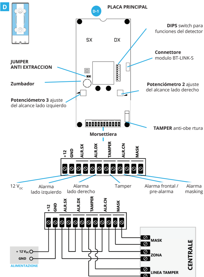
Ejemplo de conexión a una sola zona en la unidad central.
