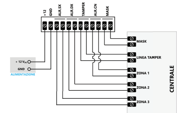
Ejemplo de conexión a tres zonas en la unidad central.
